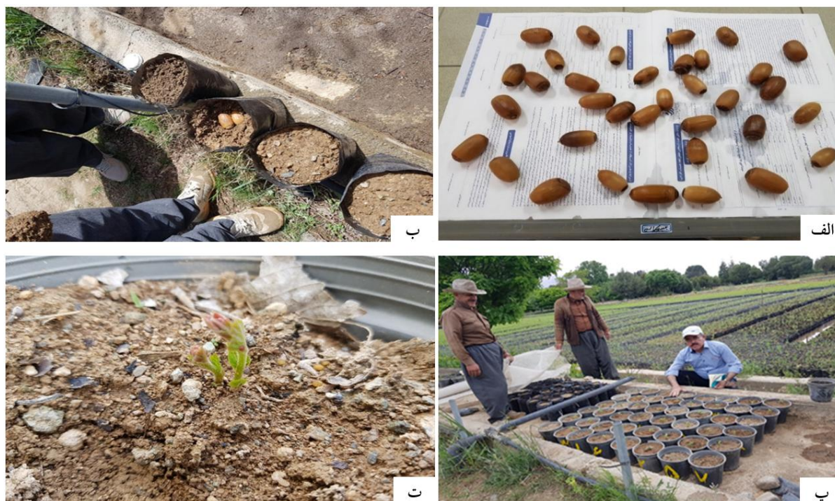
شکل ۱- الف- نمایی از خشک کردن بذور پرایم شده ب- نحوه کاشت بذر وی‌ول در گلدان پلاستیکی پ- آماده‌سازی شاسی برای چیدمان تصادفی گلدان‌ها ت- جوانه‌زنی اولین بذر و خروج گیاهچه از گلدان
